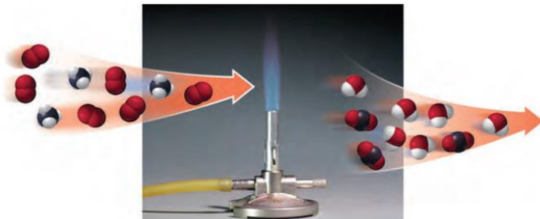
شکل ۱۶- سوختن متان. برابری شمار اتم های کربن، هیدروژن و اکسیژن در واکنش دهنده ها با فراورده ها
