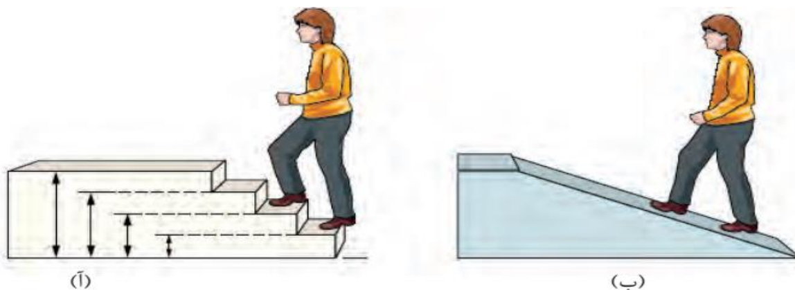
شکل ۱۹- مقایسه مصرف انرژی به صورت (آ) کوانتومی و (ب) پیوسته
