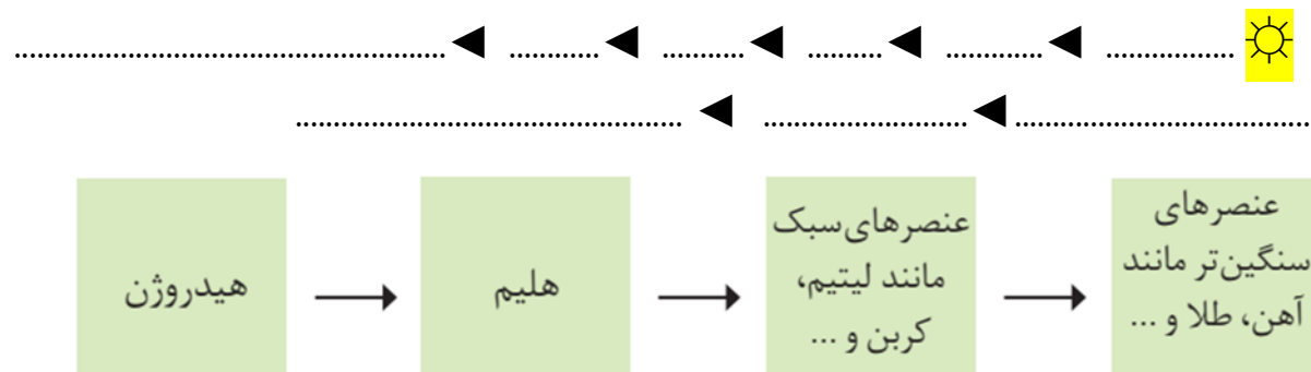
شکل ۲- روند تشکیل عناصرها
