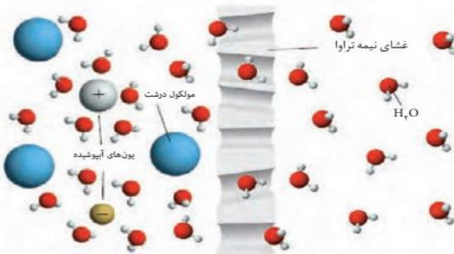
شکل ۲۶- غشای نیمه تراوا و عبور انتخابی
