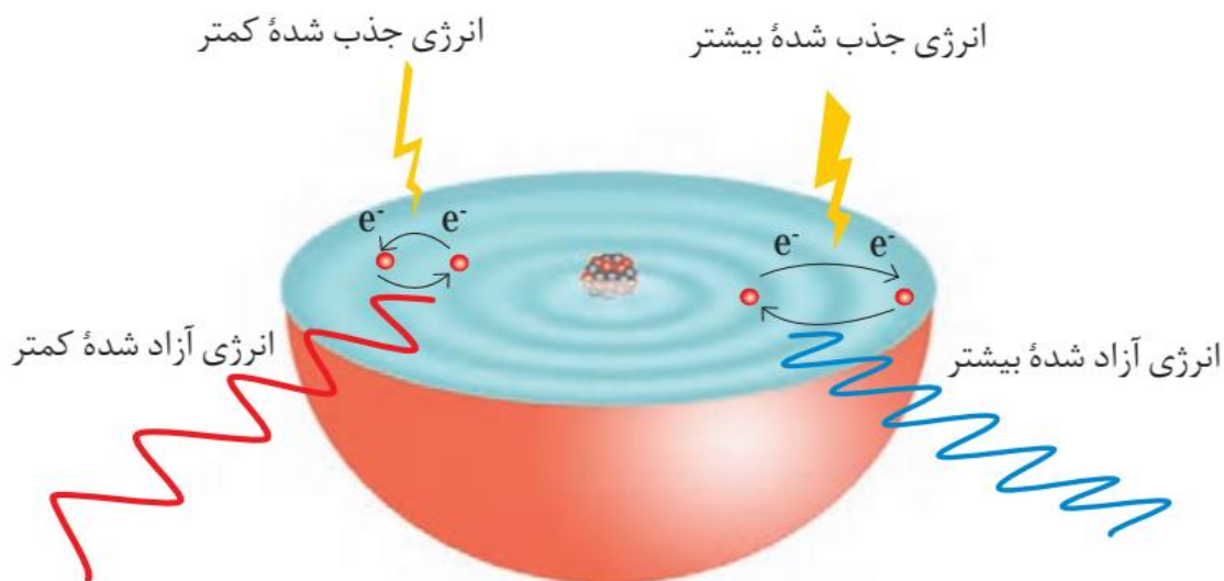
شکل ۲۰- در نتیجه جابه جایی الکترون بین لایه ها، انرژی با طول موج معین جذب یا نشر می شود.
