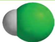
(HCl)
