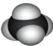
( \text{CH}_4 )
