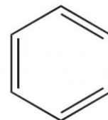
بنزن
