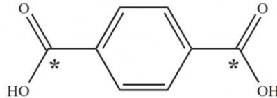
ترفتالیک اسید
