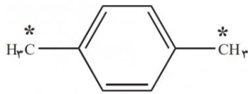
پارازایلن
