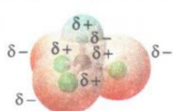
کلروفرم ( \text{CHCl}_3 )
