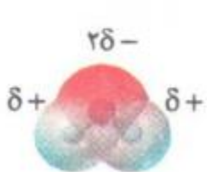
آب ( \text{H}_2\text{O} )
